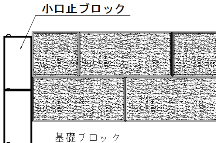
施工図
