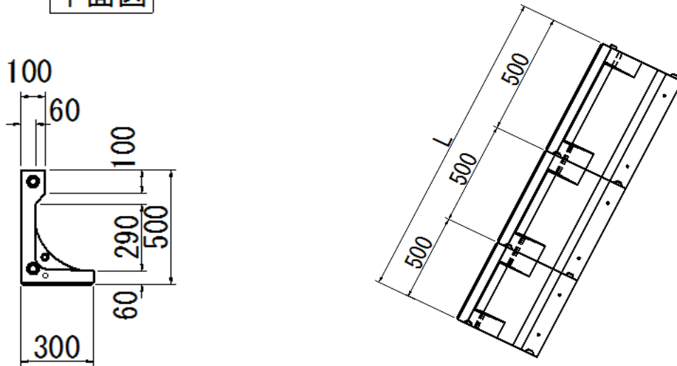
施工図
