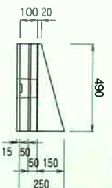
切下げ部 (歩行者用)
