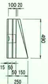
切下げ部 (車両用)
