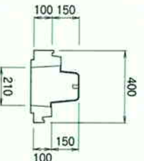
集水柵 (上部)
