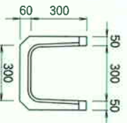
排水部 (T-25)
