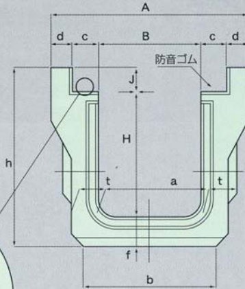
ゴム部詳細図
